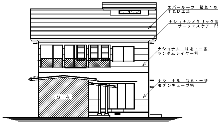
南 立 面
