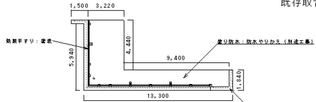
本宅 2階 防水部分
