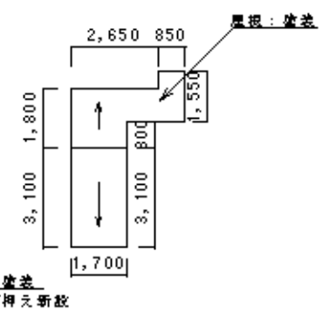
既存取合い
