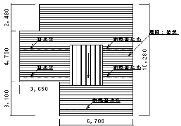
医院 横段葺き・瓦棒葺き
