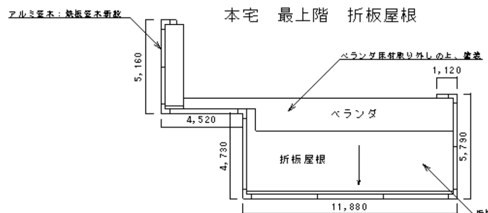
本宅 3階 折板屋根
