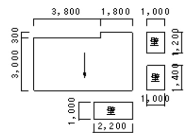
北側 ポリカ
